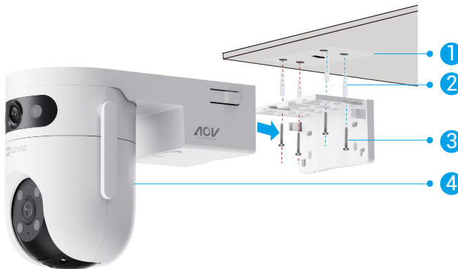
그림 1 천장 장착
