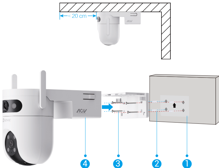
그림 2 벽 장착
